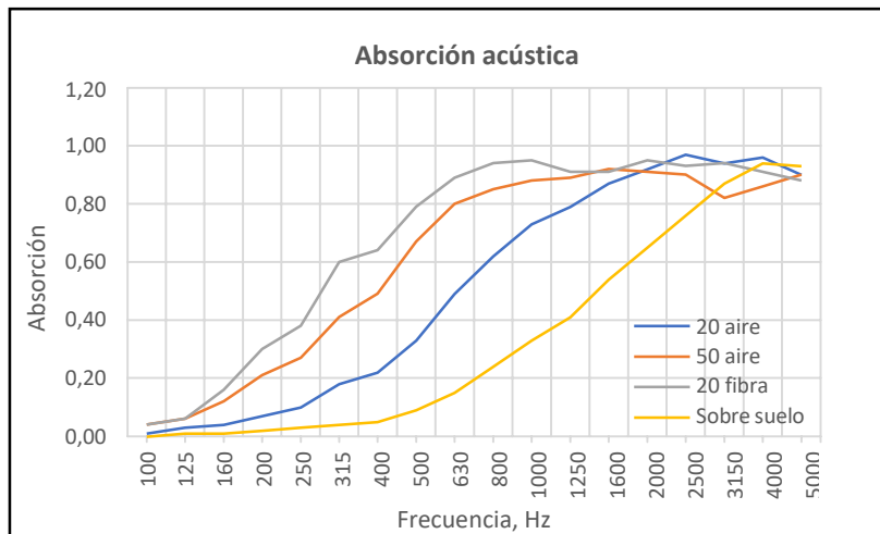
Absorción acústica de un panel Singular 12 mm espesor según normas AS ISO 354 y ASTM C453 =
